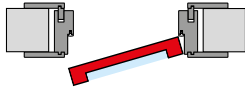
SPOSÓB MONTOWANIA SZYBY MATOWEJ (SKRZYDŁO PRAWIE – CZĘŚĆ MATOWA OD STRONY OBSERWATORA)
