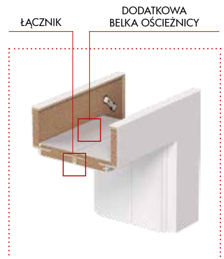
PRZEKRÓJ OŚCIEŻNICY ŁĄCZONEJ
