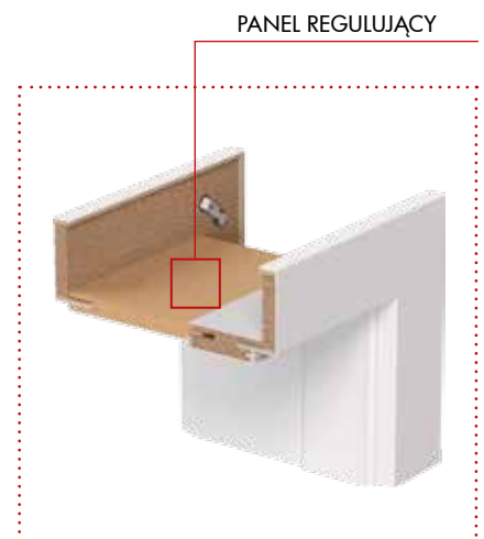
PRZEKRÓJ OŚCIEŻNICY Z PANELEM REGULUJĄCYM
