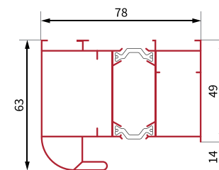
przekrój profilu ościeżnicy aluminiowej
