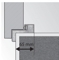
ościeznica Kątowa MAŁA PLUS
