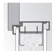
ościeznica Kątowa DUŻA montaż na ścianie kartonowo-gipsowej
