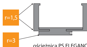
ościeżnica PS ELEGANCE dla kolekcji Porta GRANDE
