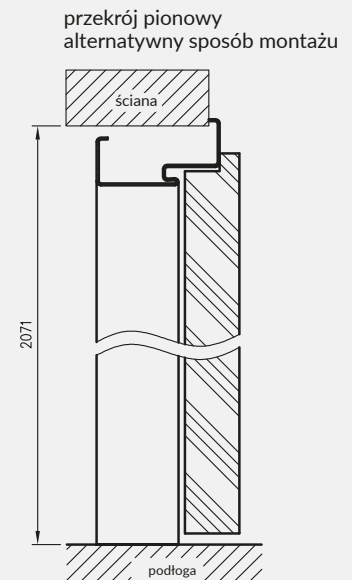
przekrój pionowy ościeżnicy stalowej stałej
