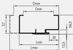
Profil ościeżnicy stalowej regulowanej z kątownikiem dymkającym T57
