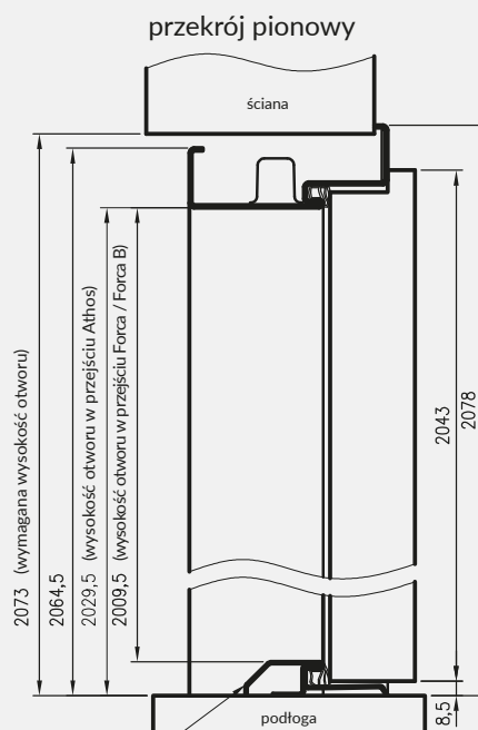
Próg stały (stalowy) do drzwi Forca i Forca B lub uszczelka opadająca w drzwiach Athos
