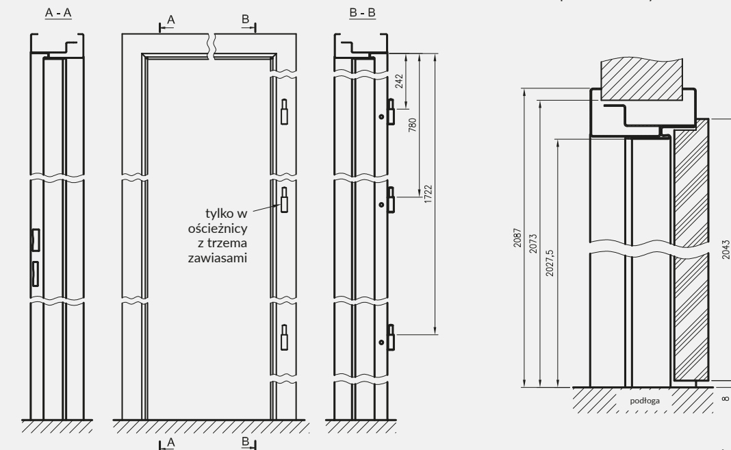
Profil ościeżnicy stalowej regulowanej z kątownikiem dymkającym T57
