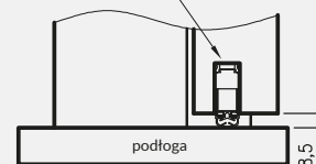
Próg stały (stalowy) do drzwi Forca i Forca B lub uszczelka opadająca w drzwiach Athos
