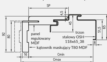
profil ościeżnicy
