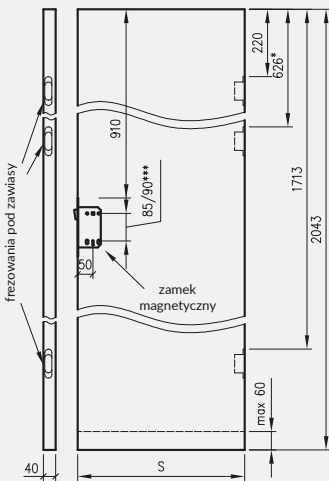
Skrzydła bezprzylgowe rozwiernie
