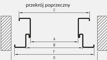
przekrój poprzeczny
