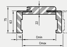
Przekrój OR/ORC z ką. T80
