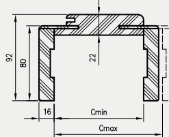
Przekrój OR/ORC z ką. T80
