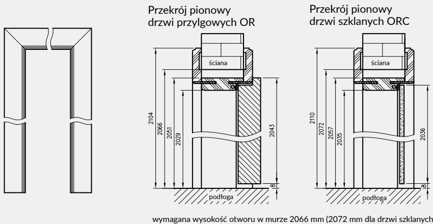
wymagana wysokość otworu w murze 2066 mm (2072 mm dla drzwi szklanych)
