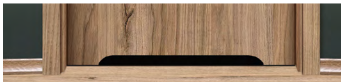
PODCIĘCIE WENTYLACYJNE INWESTYCYJNE 0,0022 m 2 (wizualizacja dla szerokości skrzydła „80”)
