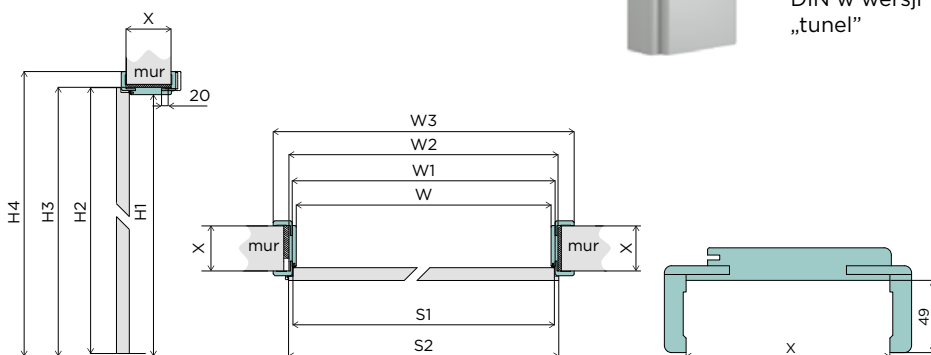
DIN w wersji „tunnel”
