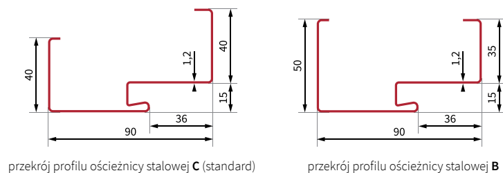
przekrój profilu ościeżnicy stalowej C (standard)
