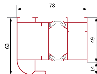
przekrój profilu ościeżnicy aluminiowej
