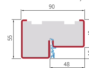
przekrój profilu ościeżnicy stalowo-drewnianej do drzwi 72 mm
