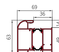
przekrój profilu ościeżnicy aluminiowej do drzwi 55 mm
