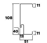
Rysunek techniczny
