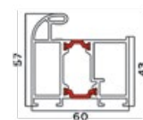
Rysunek techniczny
