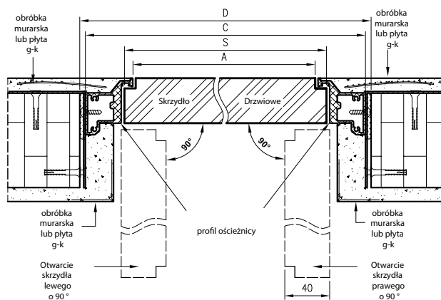
Wymiary szerokości drzwi Sara Eco 2
