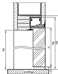
Wymiary wysokości drzwi przylgowych
