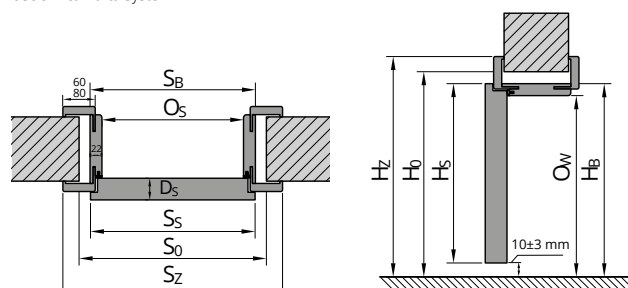
Ościeżnica Porta System
