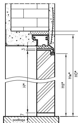
Wymiary wysokości drzwi przylgowych
