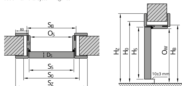
Ościeżnica Porta System Elegance
