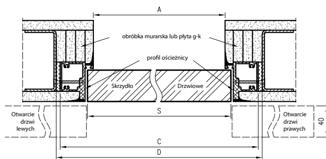
Wymiary szerokości drzwi Sara Eco 2
